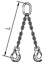
2-Strang-Anschlagkette
