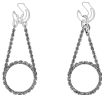
doppelt umschlungen
