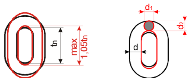
Dehnung
